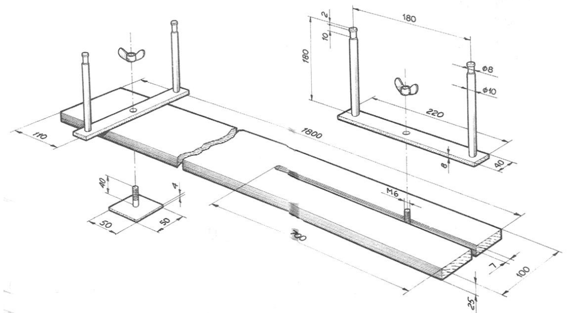
Figur 1. Konstruktion af strengbræt
